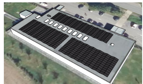
Avant-projet photovoltaïque du centre aquatique de Gouarec
